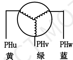
电机接线图 MOTOR WIRING DIAGRAM
